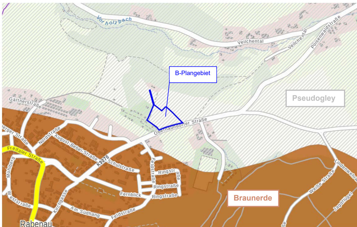
Abbildung 5: Leitbodenarten im Plangebiet – Pseudogley und Braunerde (Quelle: iDA-Portal LfULG, 19.08.2024)
